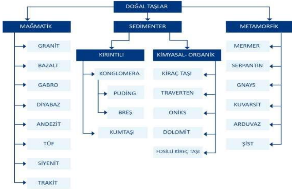
Şekil 2.3. Doğal Taşların Sınıflandırılması (Kaynak: Taşlıgil ve Şahin, 2016)
