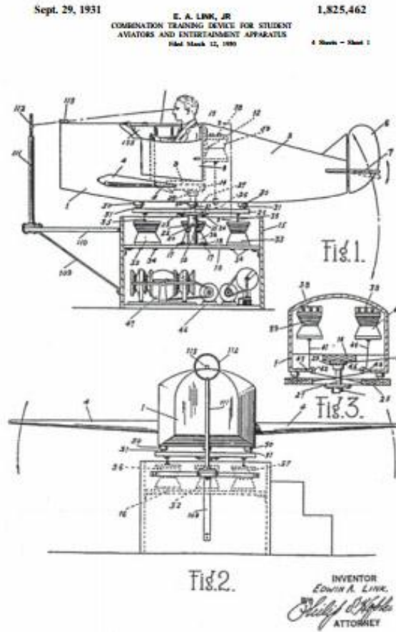
Resim 95 Edwin A. Link, Link Trainer, Orijinal patent başvuru çizimleri, 1930 208
