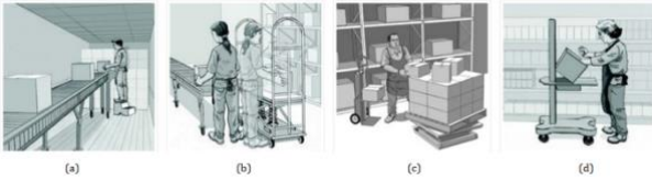
Şekil 8. NIOSH (2014) Perakende sektöründe çözüm önerileri kitapçığının ilgili görselleri (a) Kamyonun yük boşaltma ve depoya taşıma bandı; (b), (c) ve (d) ürünleri depodaki veya tezgâhtaki raflara taşıma ve yerleştirme için yüksekliği ayarlanabilen ürün taşıma arabaları
